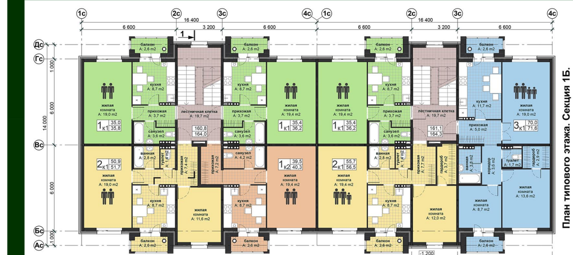
ЖИЛОЙ ДОМ. ТИП 1.
