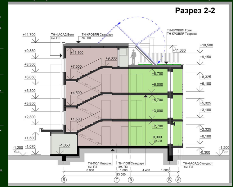
ЖИЛОЙ ДОМ. ТИП 2.
