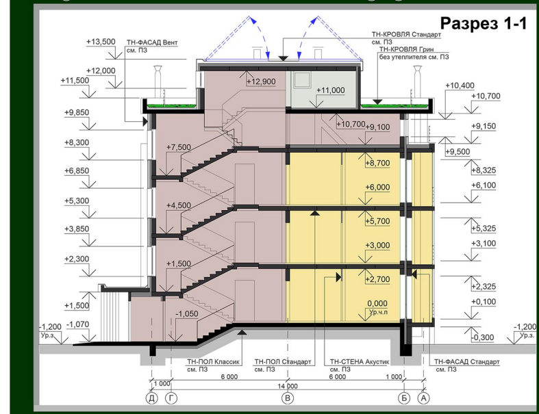
ЖИЛОЙ ДОМ. ТИП 1.
