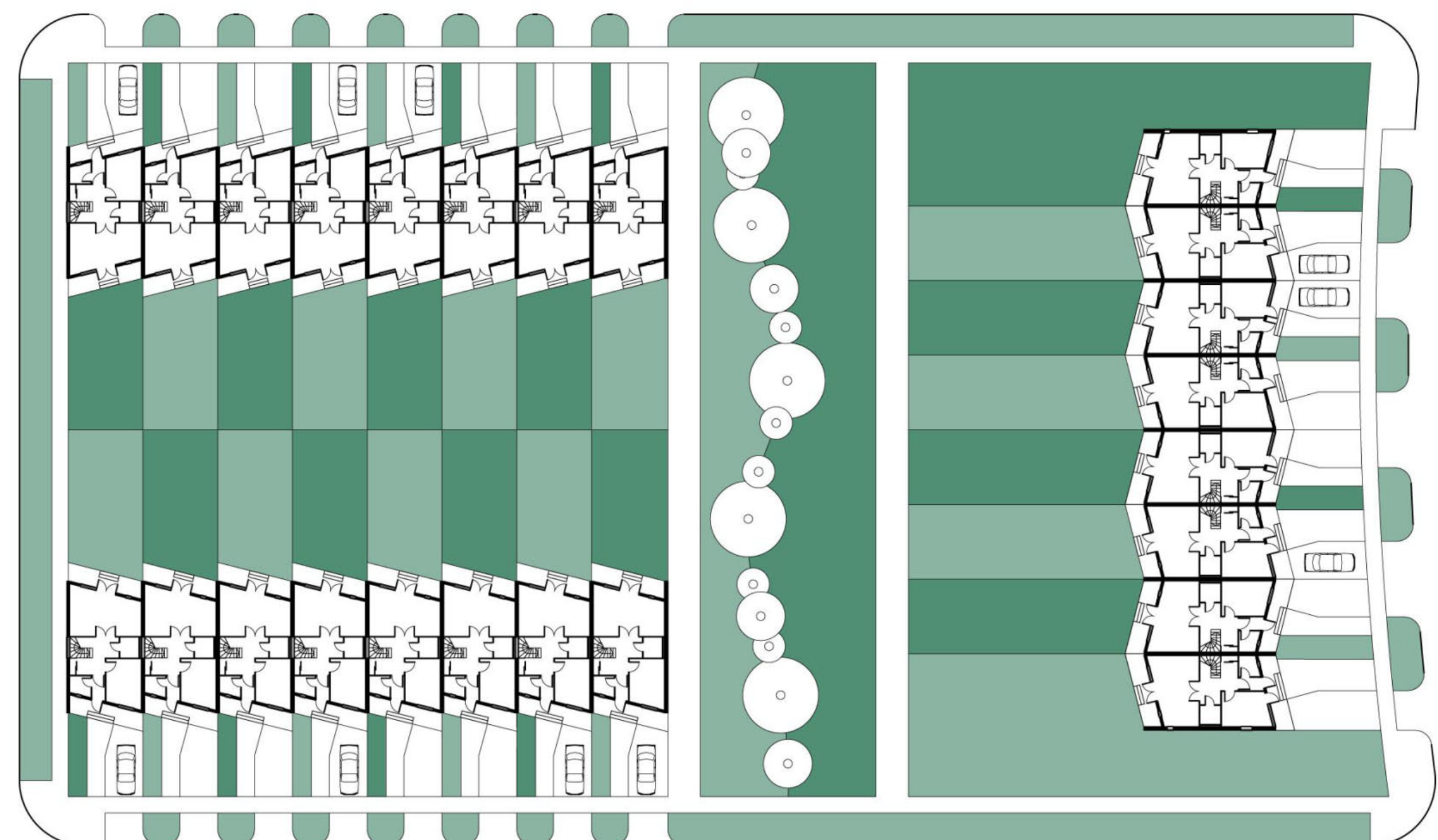
ГЕНЕРАЛЬНЫЙ ПЛАН УЧАСТКА БЛОКИРОВАННОЙ ЗАСТРОЙКИ М 1:400
