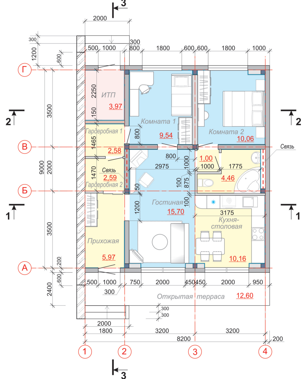
ПЛАН СЕКЦИИ 8,2x9,0. М 1:100.
