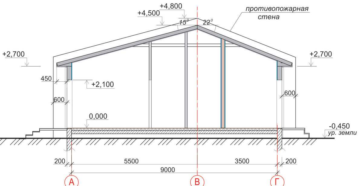
РАЗРЕЗ 3-3. М 1:100.
