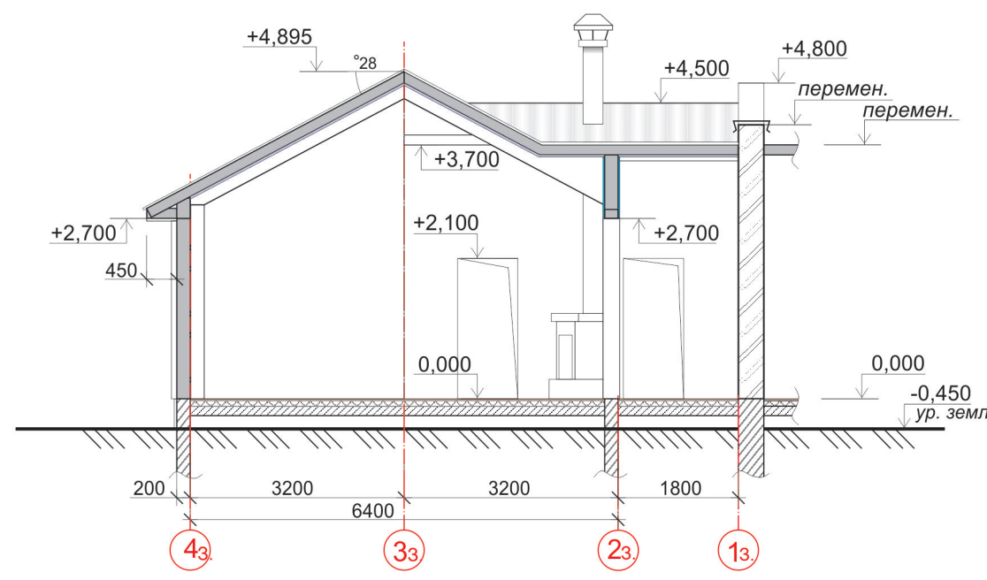
РАЗРЕЗ 2-2. М 1:100.
