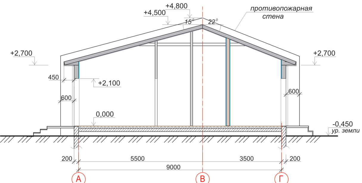
РАЗРЕЗ 3-3. М 1:100.
