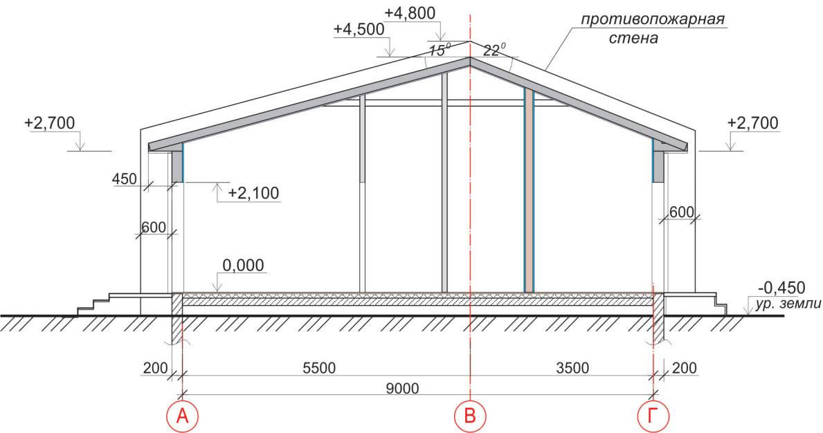
РАЗРЕЗ 3-3. М 1:100.
