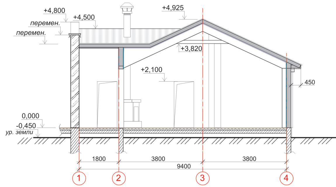
РАЗРЕЗ 2-2. М 1:100.
