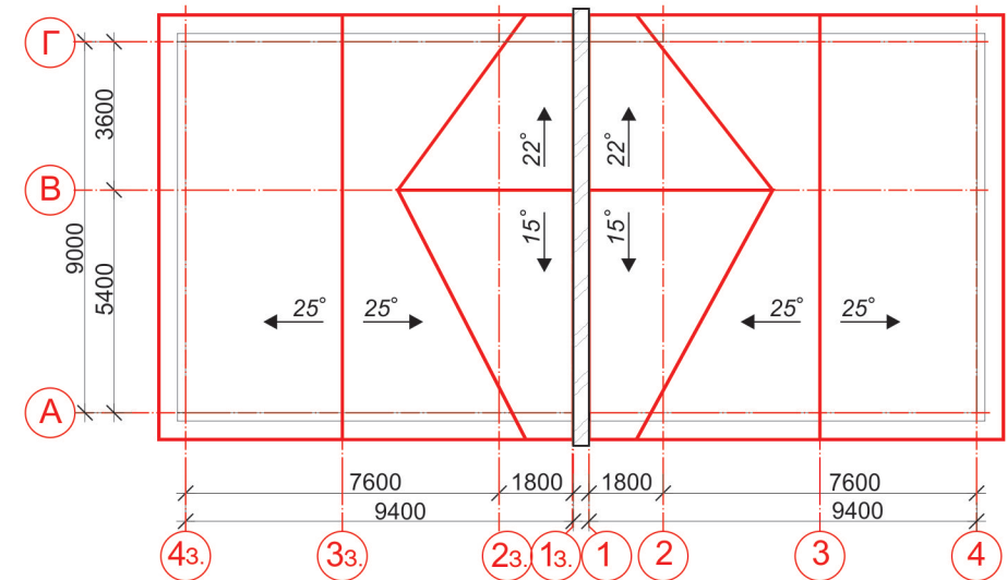
ПЛАН КРОВЛИ. М 1:200.
