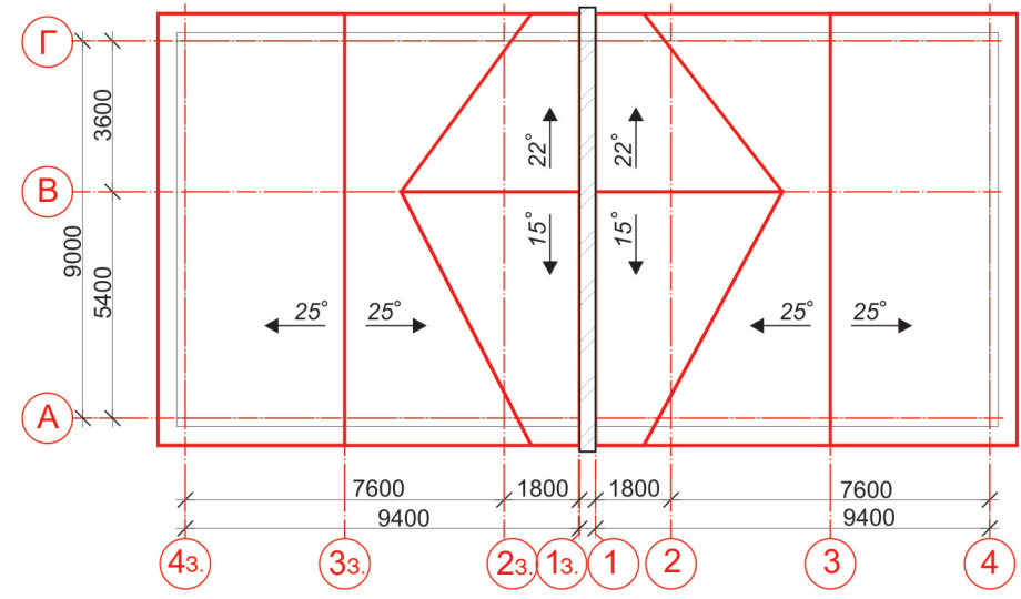
ПЛАН КРОВЛИ. М 1:200.
