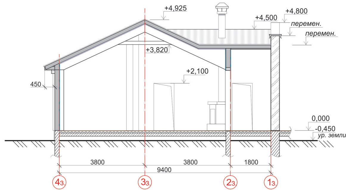
РАЗРЕЗ 2-2. М 1:100.
