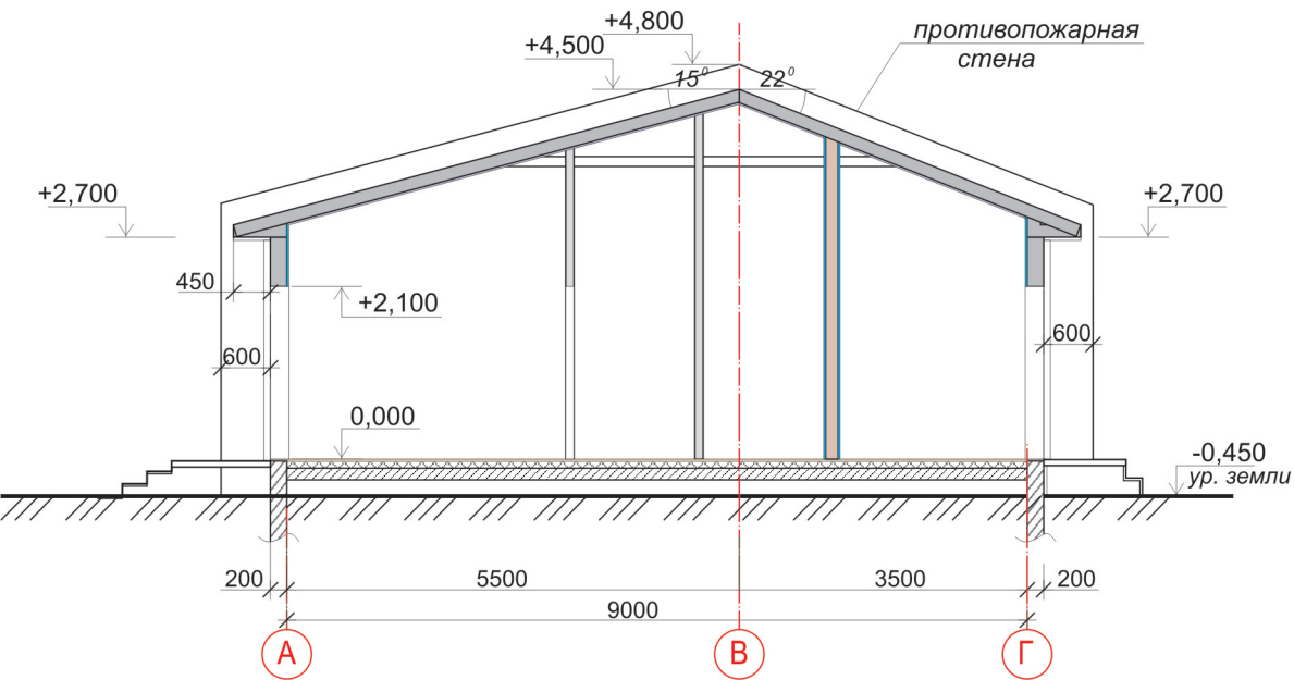
РАЗРЕЗ 3-3. М 1:100.
