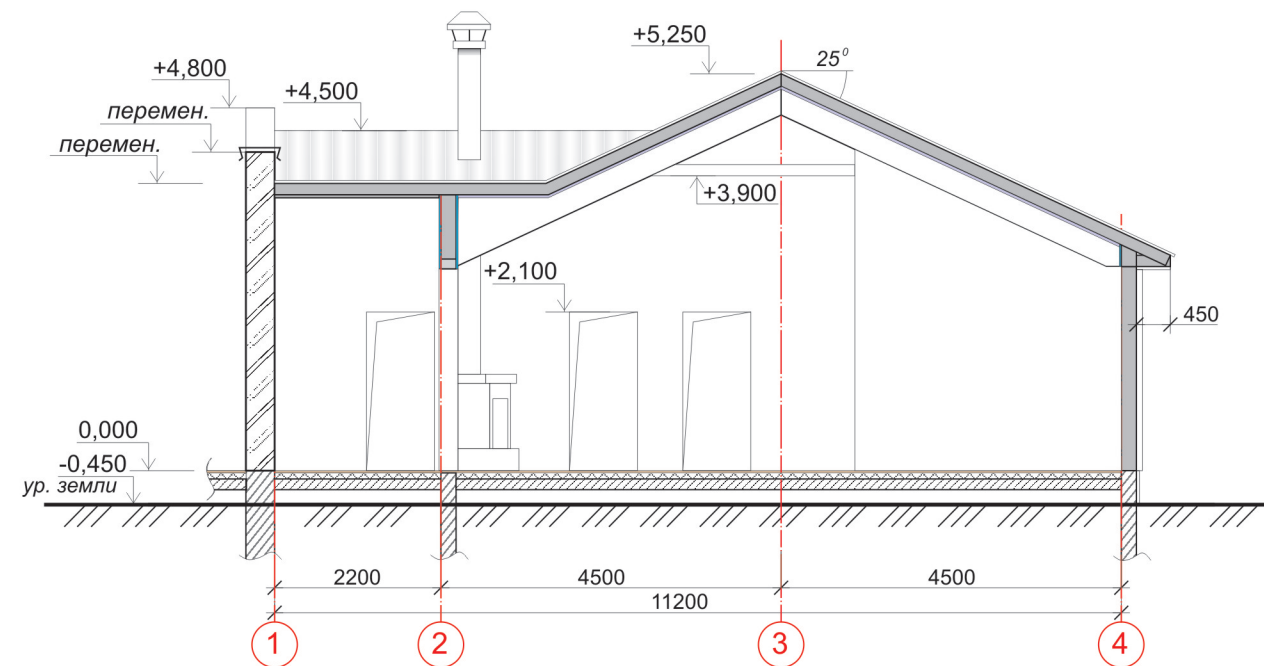
РАЗРЕЗ 1-1. М 1:100.
