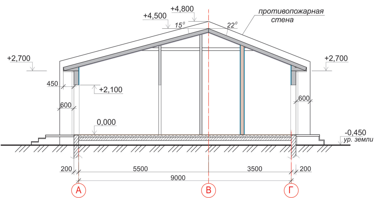
РАЗРЕЗ 3-3. М 1:100.
