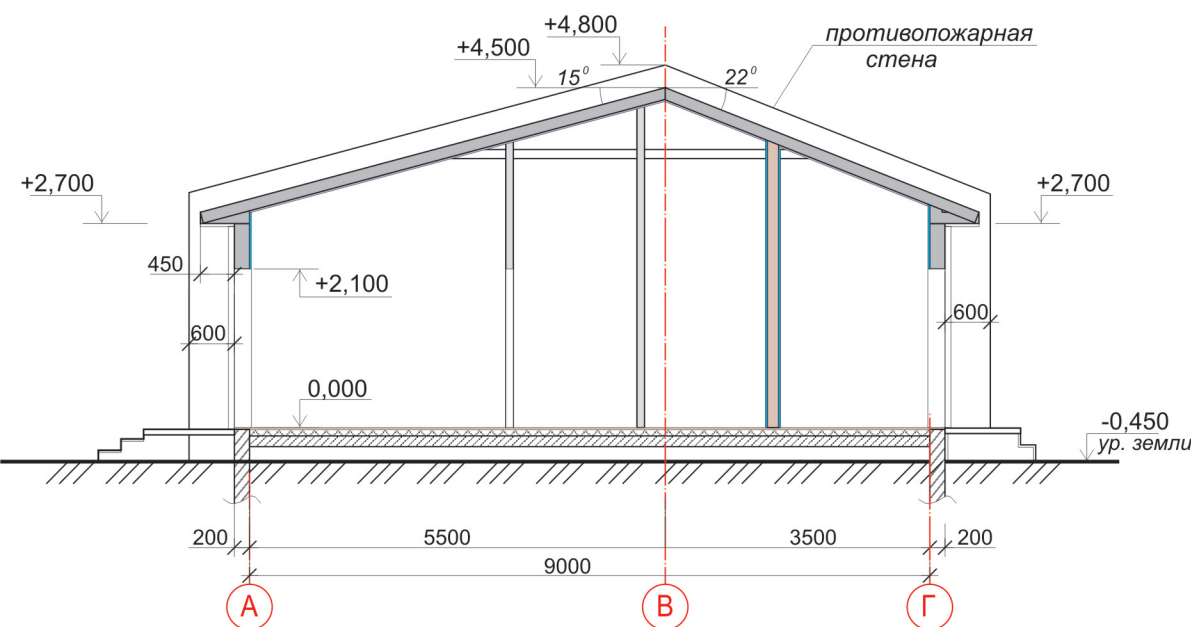
РАЗРЕЗ 3-3. М 1:100.
