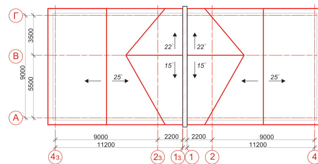
ПЛАН КРОВЛИ. М 1:200.
