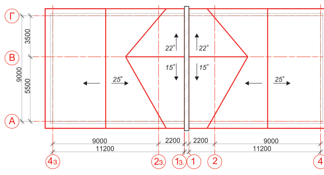
ПЛАН КРОВЛИ. М 1:200.
