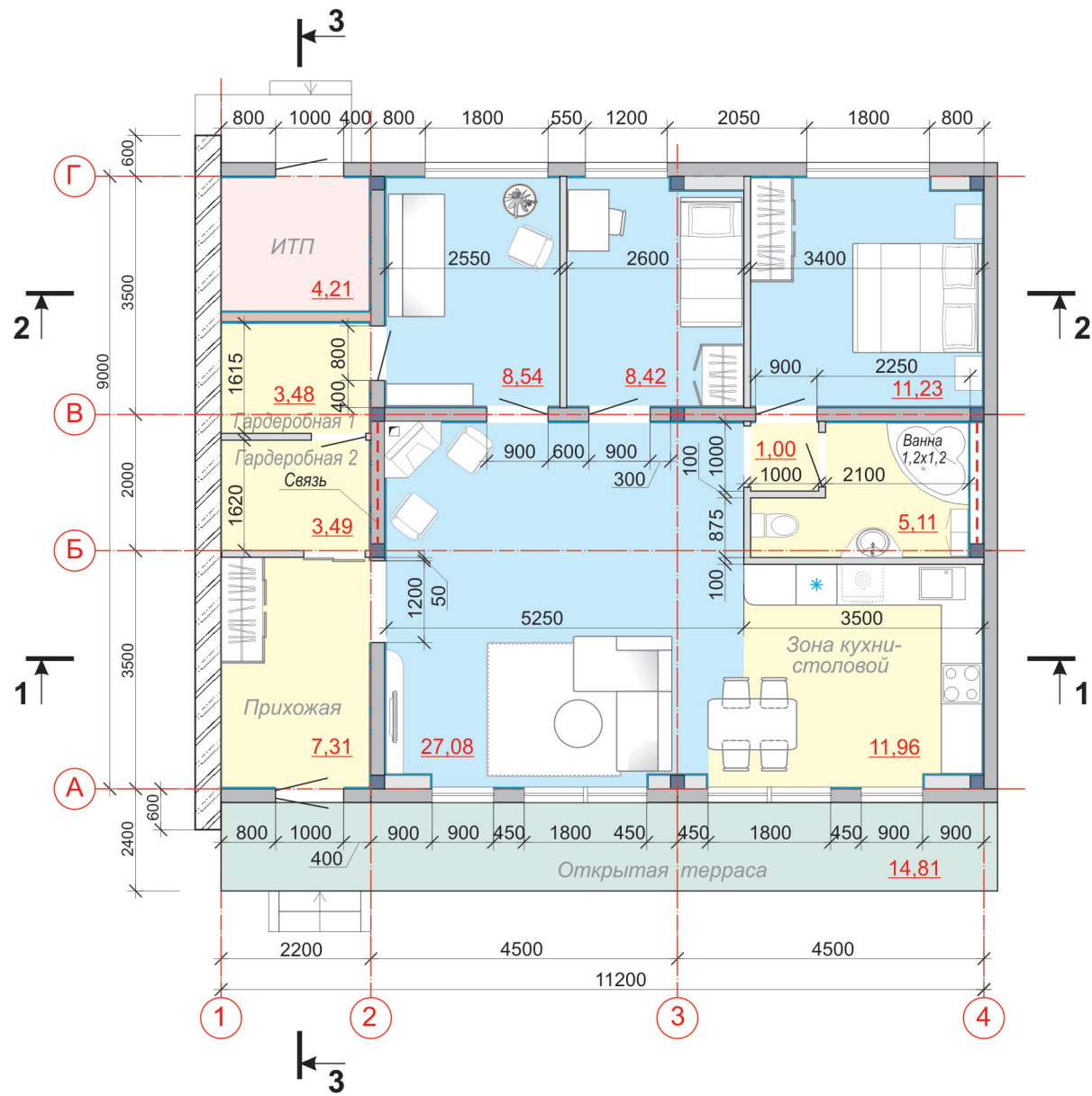
ПЛАН СЕКЦИИ. М 1:100.
