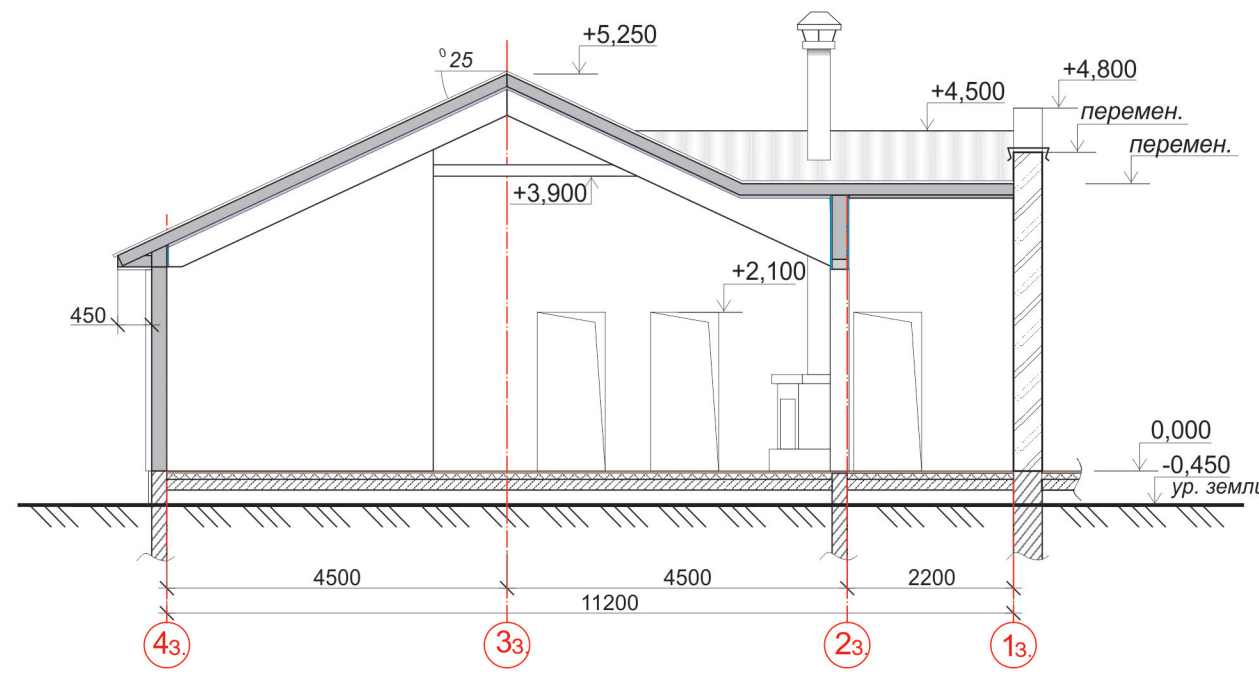
РАЗРЕЗ 2-2. М 1:100.
